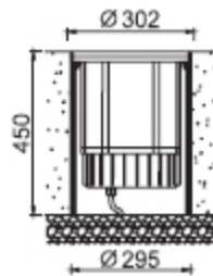
B: 250W 一体式尺寸图
